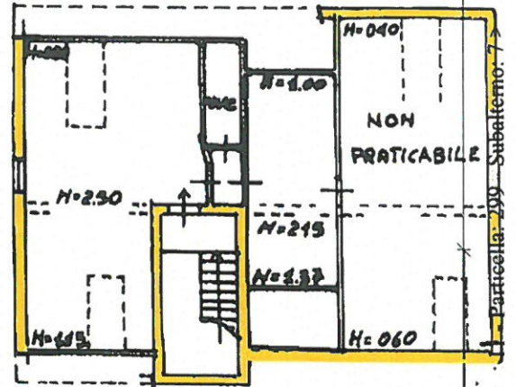
2° PIANO SOTTOTETTO
