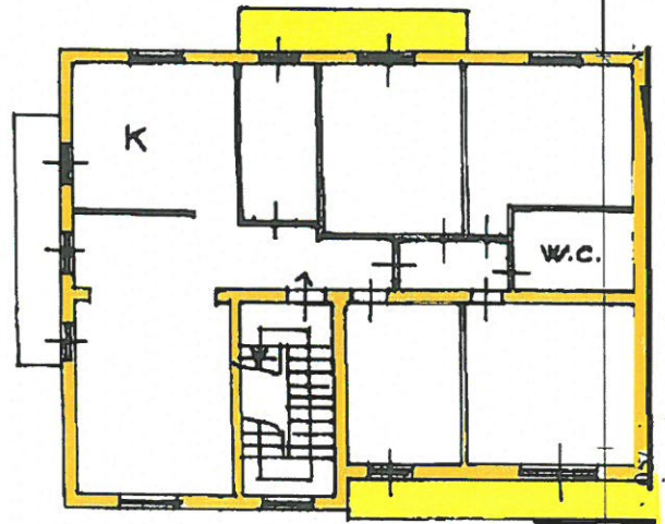
PIANO PRIMO H=3.00
