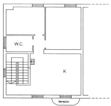
Piano Secondo h=3.00
