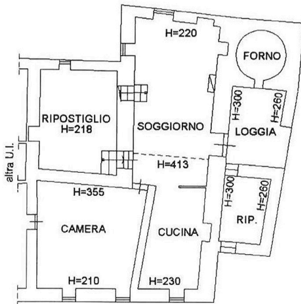
PIANO PRIMO
